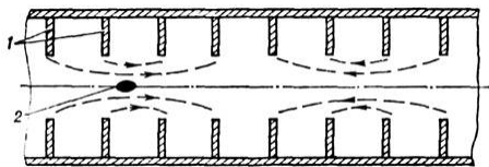
Рис. 2. Ускорение на бегущей волне: 1 - диафрагмированный волновод; 2 - ускоряемый сгусток заряженных частиц. Стрелками показано распределение напряжённости электрического поля, бегущего вдоль волновода.
