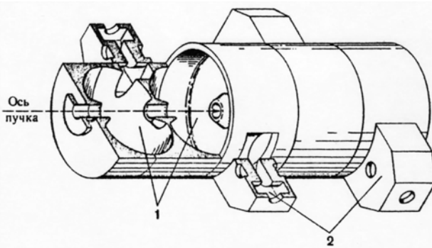
Рис. 4. Система с боковыми резонаторами связи. Форма ускоряющих резонаторов подобрана так, чтобы параллельное сопротивление системы было максимальным. Для уменьшения вносимой щелями асимметрии резонаторы связи расположены попеременно с разных сторон системы. 1 – ускоряющие резонаторы; 2 – резонаторы связи.
