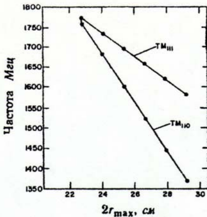
Рис. 16. Зависимость частот поперечных типов колебаний от r_{\max} для резонаторов с \beta = 0,65 .
