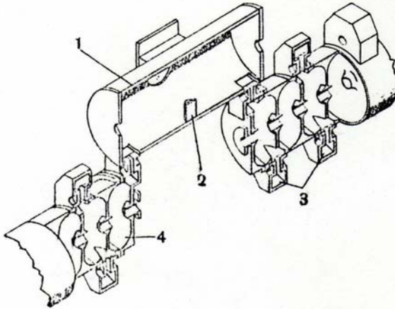
Рис. 18. Геометрия соединительного устройства, введенного в секцию K . 1 – соединительный резонатор; 2 – резонансный штырь; 3 – резонаторы связи; 4 – ускоряющий резонатор,
