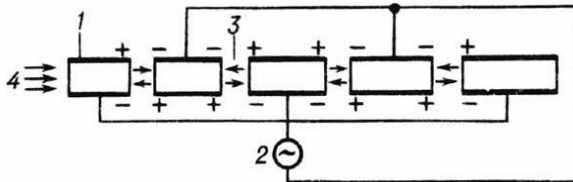
Рис. 1. Принципиальная схема ускорителя с пролетными трубками: 1 - пролетные трубки; 2-генератор ВЧ-колебаний; 3- ускоряющие зазоры; 4- источник частиц.
