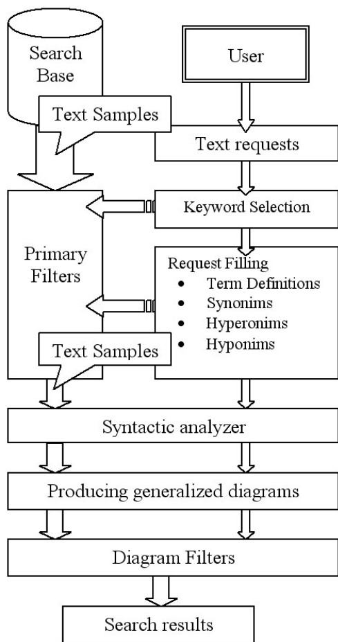
Рис. 2. Схема поискового ядра системы iNetSearch
