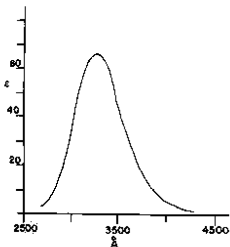
Рис. V-16. Коэффициенты поглощения \text{Cl}_2 в области 2500 – 4500 Å [393]. Коэффициент \epsilon выражен в л/ (моль · см), основание 10, температура комнатная. [Copyright, 1933 by the American Institute of Physics.]
